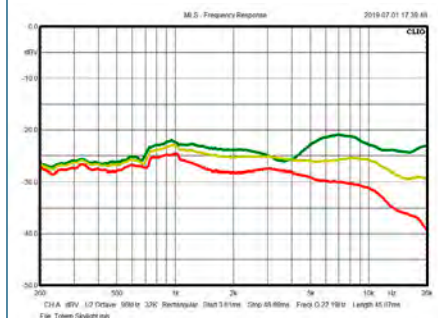
Med tanke på ljudet har Totem lite oväntat gropig frekvens framifrån (grön). Vid 30 grader (gul) är det lite bättre. Fallet vid 60 grader (röd) är också hyggligt jämnt, och bör därmed inte vinklas så mycket mot lyssnaren.
