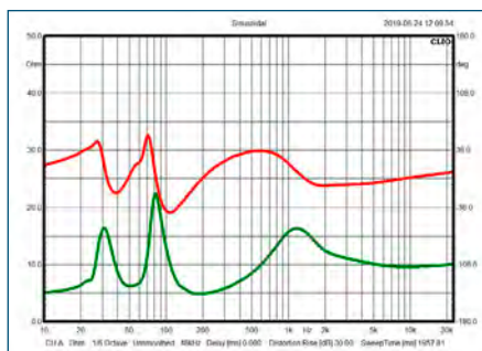
Med sina 84 dB (på pappret) är Dynaudio visserligen lite effekt-krävande, men impedansen (grön) är rätt harmlös. Aldrig under 5 ohm. Fasnörelserna (röd) kunde varit mjukare i basen.
