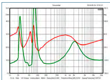
Inte heller Totem är helt snäll mot förstärkaren. Impedansen (grön) går visserligen aldrig under 6 ohm, men fasväxlingarna (röd) i basen är lite väl skarpa.
