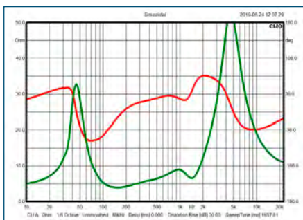
Arendals impedans (grön) går visserligen aldrig under 4 ohm, men svajig fas (röd) och känslighet på låga 84 dB gör den till en krävande last.
