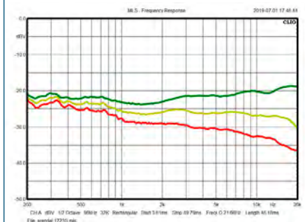
Arendal har mycket fin linjäritet. Framifrån (grön) finns en svag diskantshöjning som blir en svag men jämn nivå-sänkning vid 30 grader (gul). Tydligare vid 60 grader (röd).
