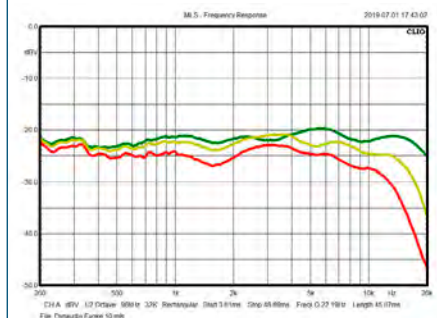
Dynaudio har hyggligt jämn frekvens mätt framifrån (grön), men tydligt diskantfall vid 30 grader (grön), som blir brantare vid 60 grader (röd).
